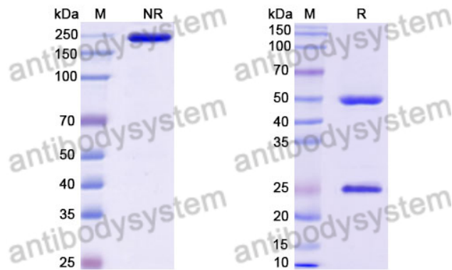
SDS PAGE for Raludotatug
