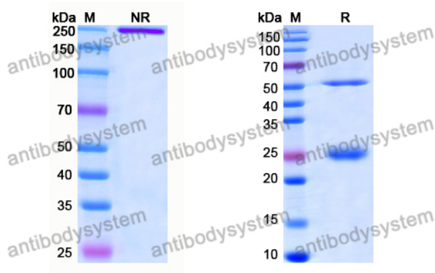
SDS-PAGE
