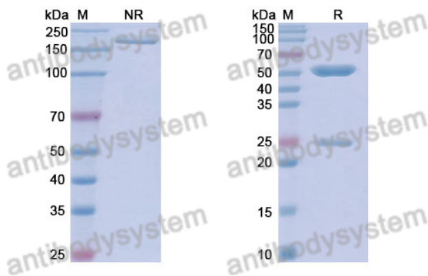
SDS-PAGE
