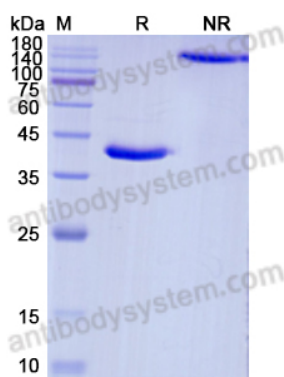
SDS-PAGE
