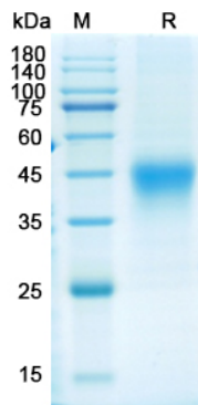
SDS-PAGE
