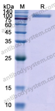
SDS-PAGE
